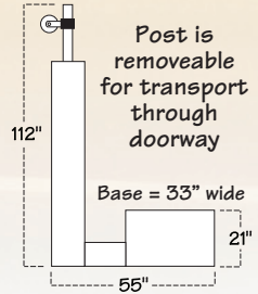
Wormgear Net Tensioning Crank
